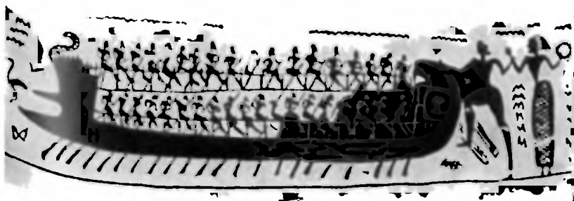
Пятидесятивесельный корабль.
