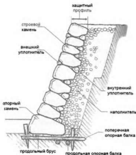
Профиль каменной стены
