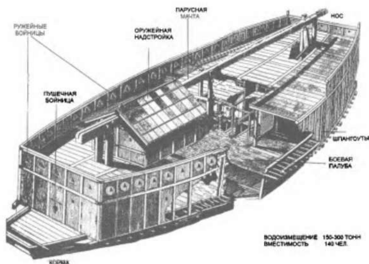
Боевая ладья XVI века (флот Мори)
