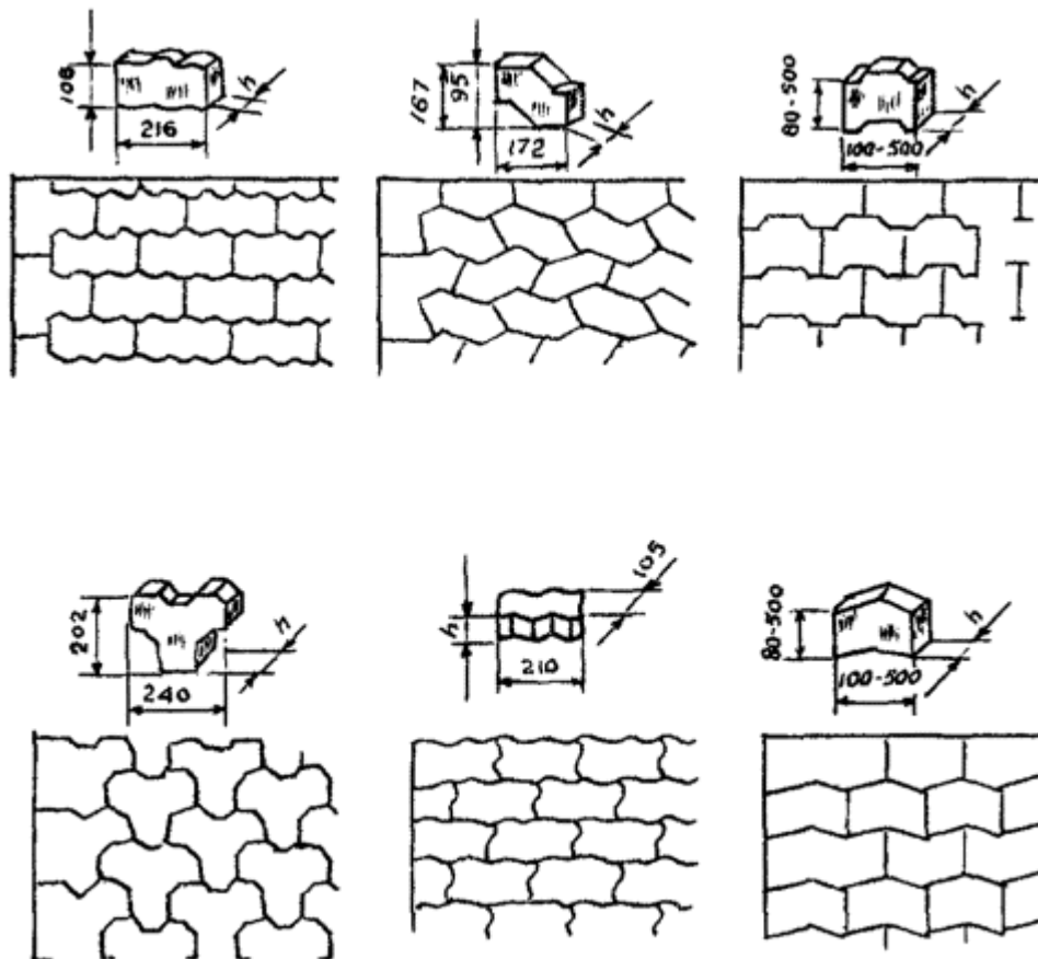
Рис. 4. Типы и схемы раскладки фигурных элементов мощения.
