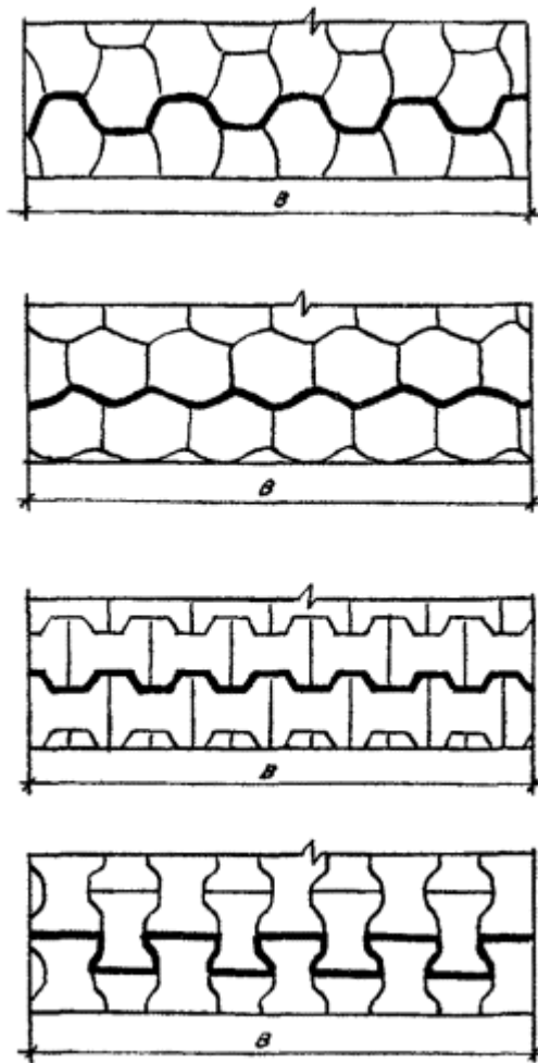
Рис. 5. Расположение швов расширения в покрытии тротуара.
